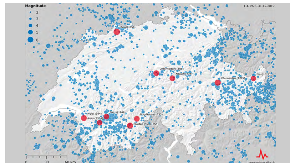
Sismicité de la Suisse et des zones alentours entre avril 1975 et fin 2019 (en bleu), ainsi que l'épicentre des dix plus puissants séismes connus dans l'histoire (en rouge). Source : Service Sismologique Suisse, 2020.
